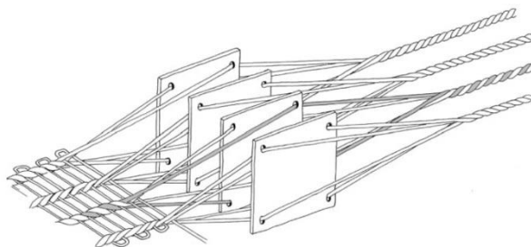
Fig. 1 - Ricostruzione della tecnica produttiva della tessitura a tavolette (Ræder Knudsen 2012, fig. 11.1).
