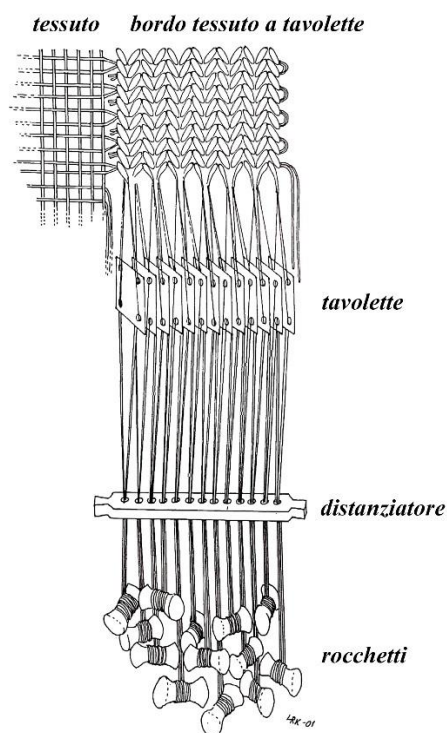
Fig. 2 - Ricostruzione della tecnica produttiva di un bordo tessuto a tavolette con rocchetti (von Eles 2019, fig. 2.1.2).
